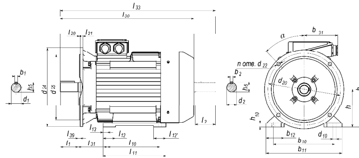
Привязка мощностей к установочно - присоединительным размерам по стандартам ГОСТ 31606 Power binding to mounting and overall dimensions according to GOST 31606
