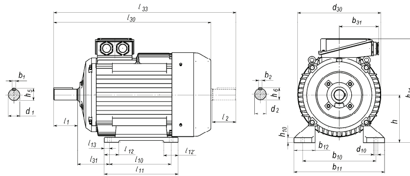
Привязка мощностей к установочно - присоединительным размерам по стандартам DIN EN 50347 Power binding to mounting and overall dimensions in according to DIN EN 50347
