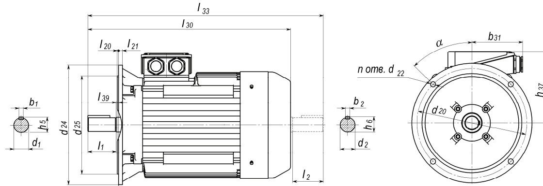
Привязка мощностей к установочно - присоединительным размерам по стандартам DIN EN 50347 Power binding to mounting and overall dimensions according to DIN EN 50347
