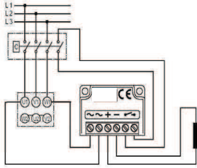
Схема подключения от контактов в коробке выводов двигателя. Не доустима при работе от преобразователя частоты
