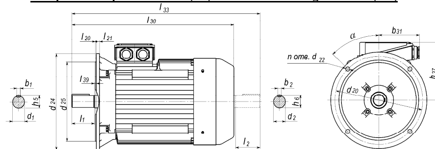
Привязка мощностей к установочно - присоединительным размерам по стандартам ГОСТ 31606 Power binding to mounting and overall dimensions according to GOST 31606
