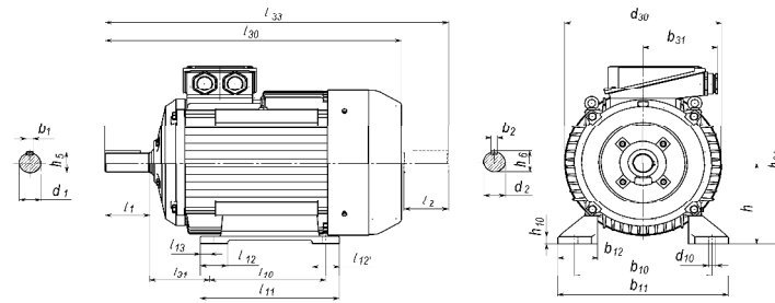
Привязка мощностей к установочно - присоединительным размерам по стандартам ГОСТ 31606 Power binding to mounting and overall dimensions according to GOST 31606
