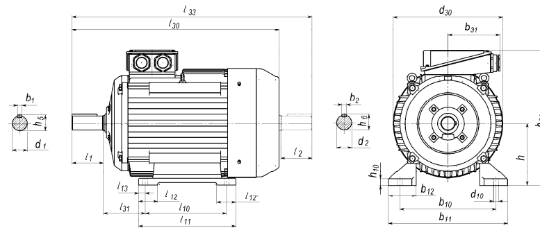
Привязка мощностей к установочно - присоединительным размерам по стандартам ГОСТ 31606 Power binding to mounting and overall dimensions according to GOST 31606 Размеры в мм / Dimensions in mm
