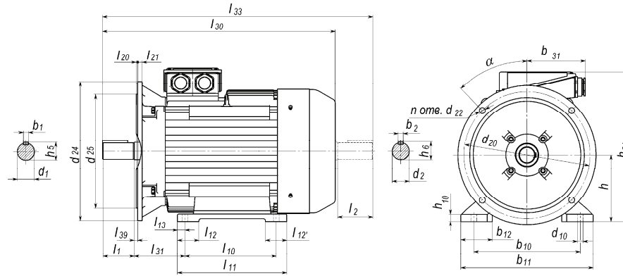
Привязка мощностей к установочно - присоединительным размерам по стандартам DIN EN 50347 Power binding to mounting and overall dimensions according to DIN EN 50347
